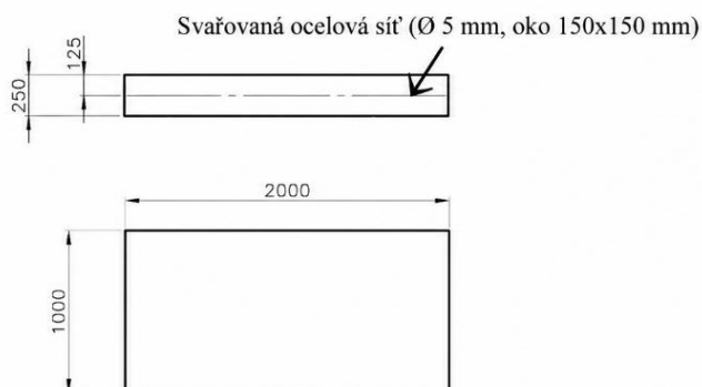
Železobetonový základ, TAU TUBE P50
