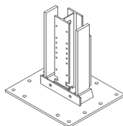
Zadní konzola (kód č.0080)
